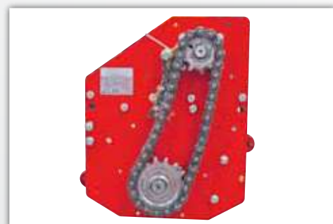
Transmisión lateral de cadena en baño de aceite (modelo "L")
